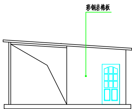
侧立面图
